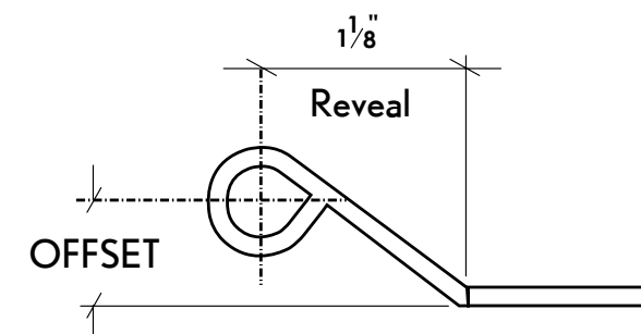
HINGE
