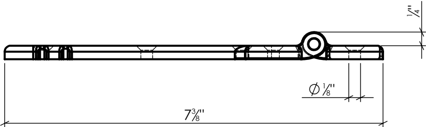
'L' Hinge
