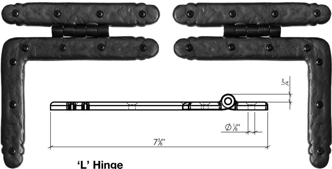
'L' Hinge
