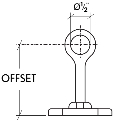
PINTLE
