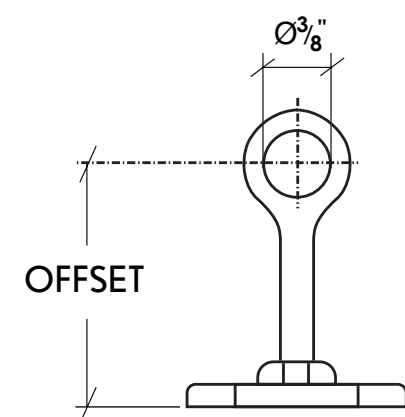
PINTLE
